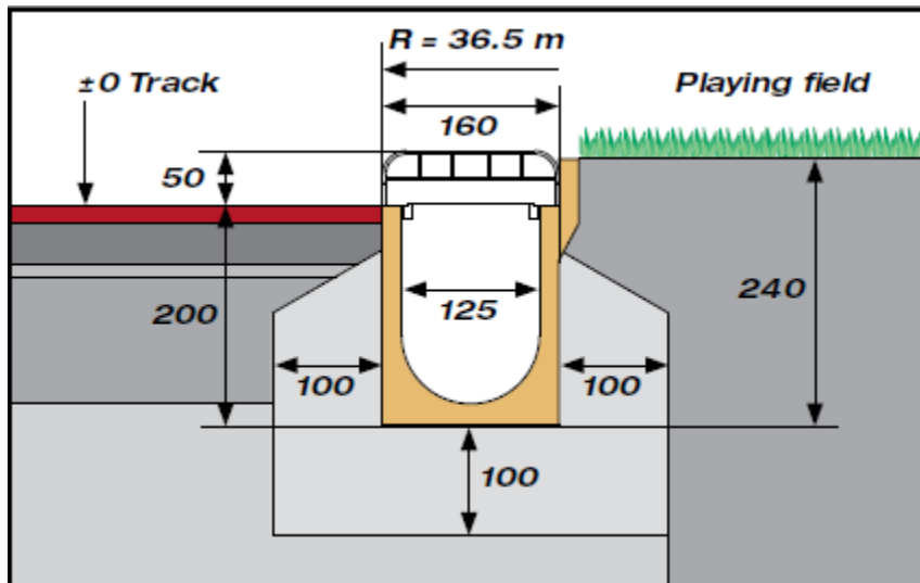
ANRIN sportrennid 125- E/F, sirged ja raadiusega, plastikrestiga
